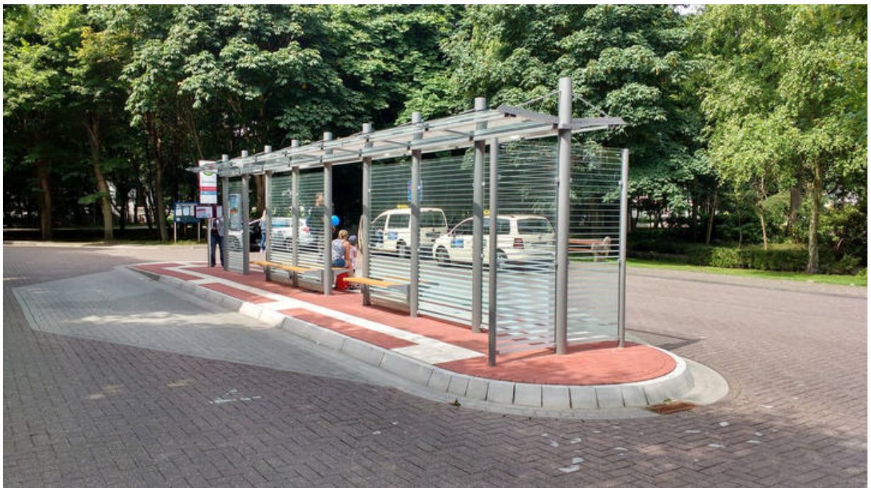
Warteinsel am Rosengarten mit doppelzeiliger Wartehalle System O
