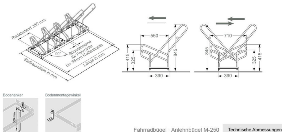
Abmessungen Anlehnparker M-250
