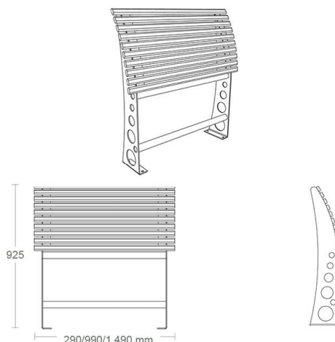
Anlehnbank LEAN mit Alu-Vollprofilen Technische Abmessungen
