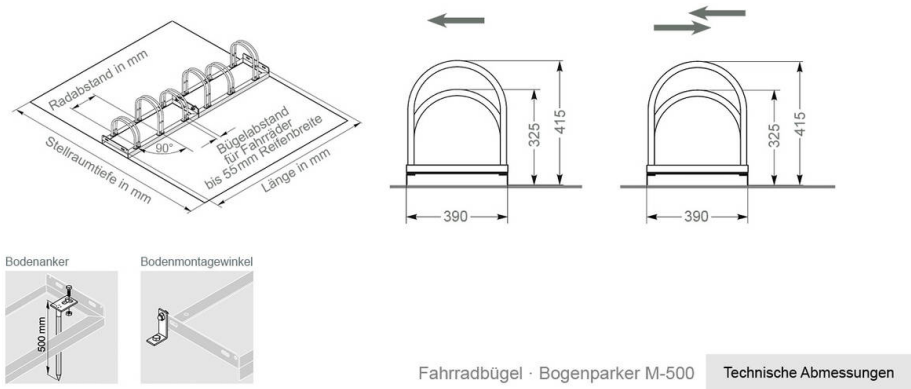
Abmessungen Bogenparker M-500
