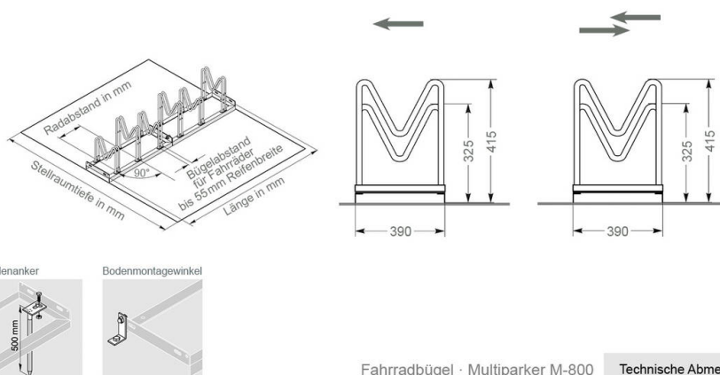
Abmessungen Multiparker M-800
