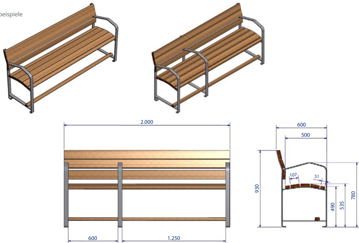
Seniorenstuhlsbank TESS2 in V2A (2.000 mm) mit Zusatzelement Armlehne und Fußstütze
