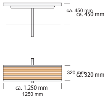
Sitzbank Typ L (einzell) für 2 Personen (in RAL 9006 Weißaluminium)
