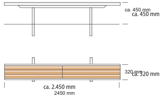
Sitzbank Typ L (doppel) für 4 Personen (in RAL 9006 Weißaluminium)
