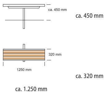
Sitzbank Typ L (einzeln) für 2 Personen (in RAL 9006 Weißaluminium)
