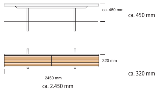
Sitzbank Typ L (doppel) für 4 Personen (in RAL 9006 Weißaluminium)
